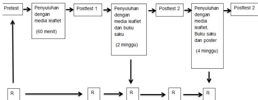
Gambar 3. Kerangka Penelitian
