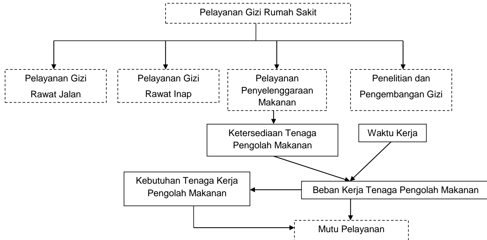
Gambar. 2 Kerangka Konsep
