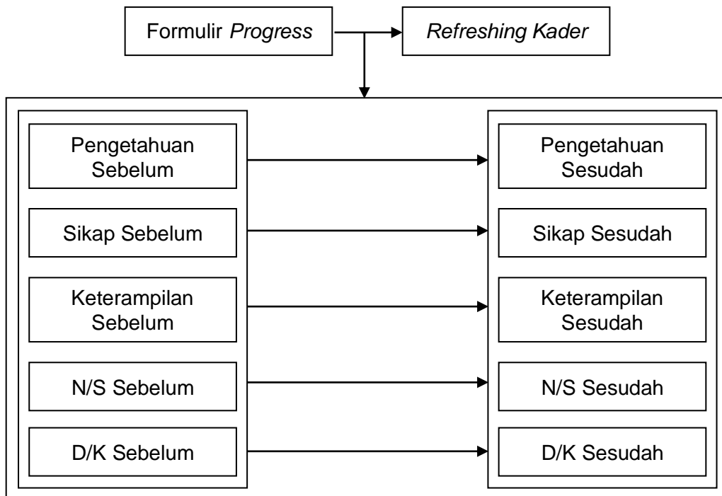
Gambar 1. Kerangka Konsep
