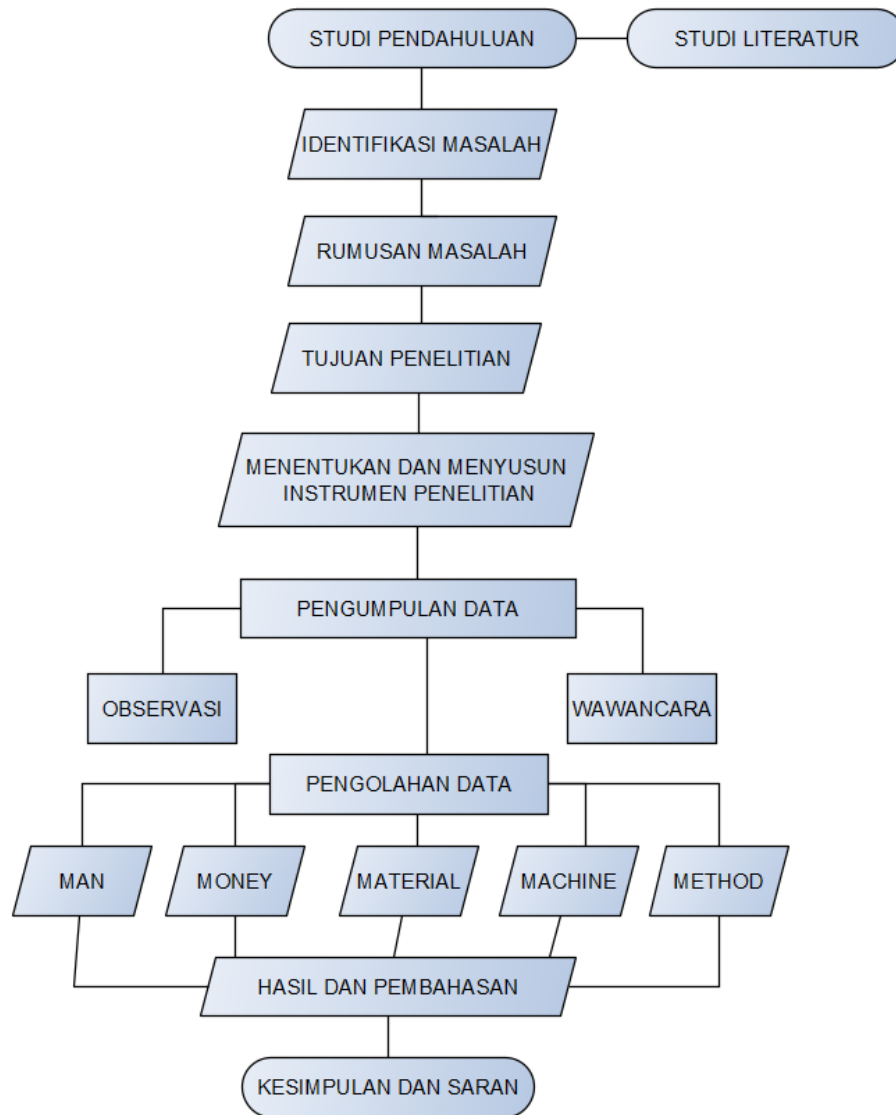
Gambar 3.1 Tahap Penelitian
