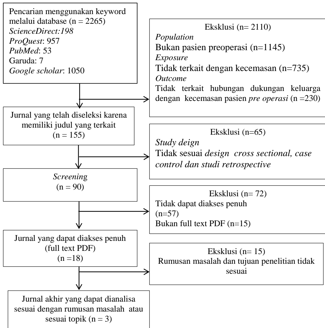
Gambar 3. 1 Diagram Flow PRISMA Hasil Pencarian dan Seleksi Studi
